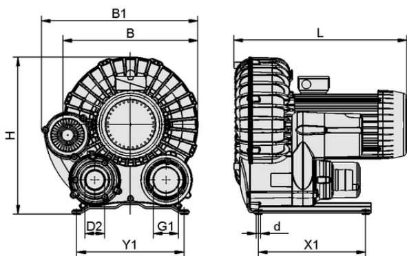
Datos de diseño SB 325 265 3 IE3-TYP3
