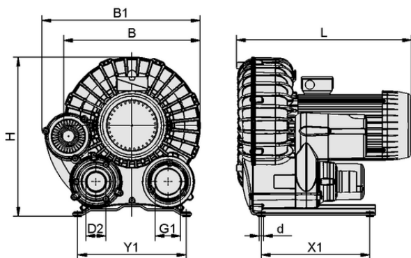
Données de construction SB 180 215 1.5 IE3-TYP3
