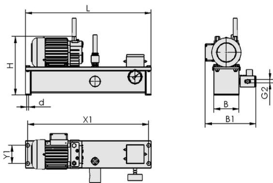
Données de construction VZ-TR 4 AC 5 IE3-TYP1
