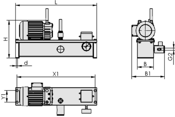
Tasarım verileri VZ-TR 4 AC 5 IE3-TYP1
