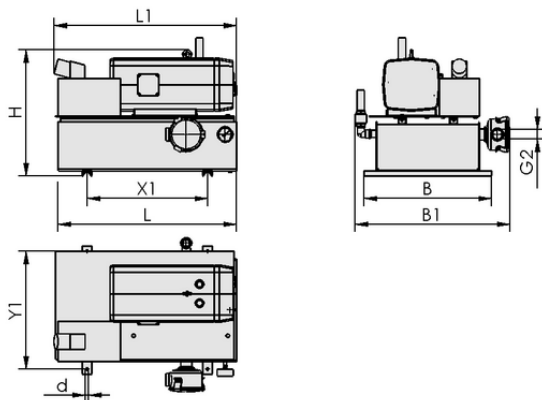
Dati di costruzione VZ-TR 80 AC3 100 MS IE3-TYP1
