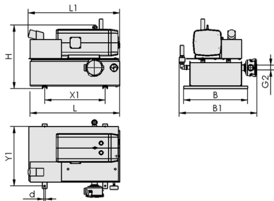
デザインデータ VZ-TR 80 AC3 100 MS IE3-TYP1
