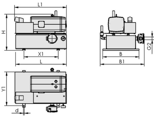
Données de construction VZ-OG 165 AC3 200 MS
