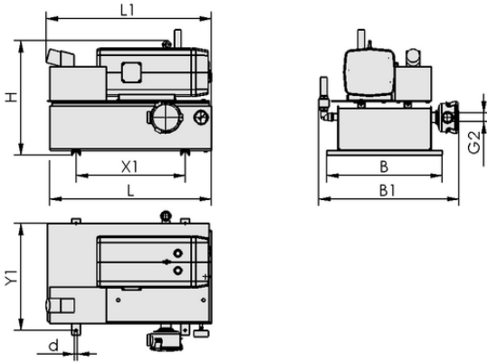
Tasarım verileri VZ-OG 165 AC3 200
