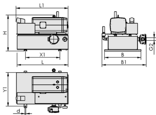
Données de construction VZ-OG 100 AC3 100 MS
