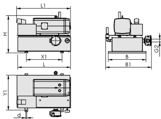
デザインデータ VZ-TR 25 AC3 50 MS
