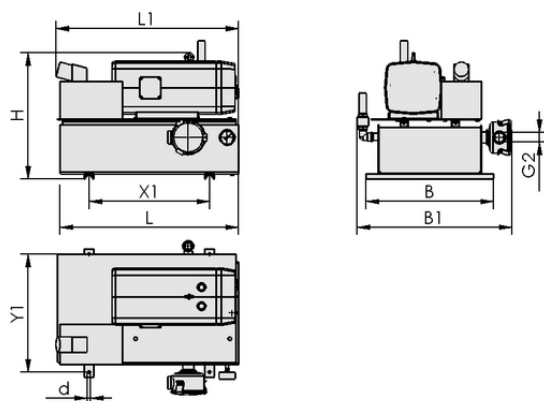
Données de construction VZ-OG 63 AC3 100
