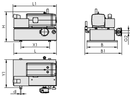
Dati di costruzione VZ-OG 63 AC3 100
