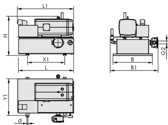
Données de construction VZ-OG 100 AC3 100 GMS
