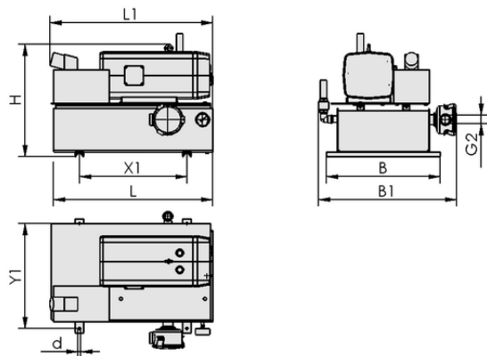
Dati di costruzione VZ-TR 25 AC3 50 GMS
