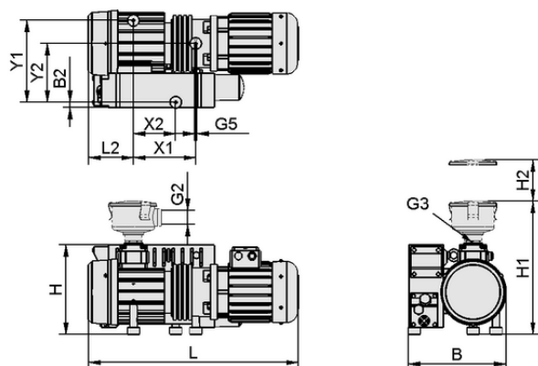
Dati di costruzione EVE-OG 10 AC3 F
