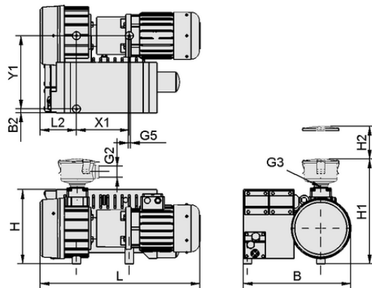
Konstruktionsdaten EVE-OG 63 AC3 AQUA IE2
