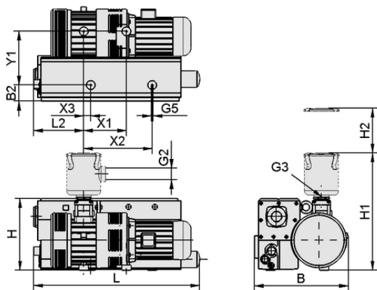
Dati di costruzione EVE-OG 255 AC3 F
