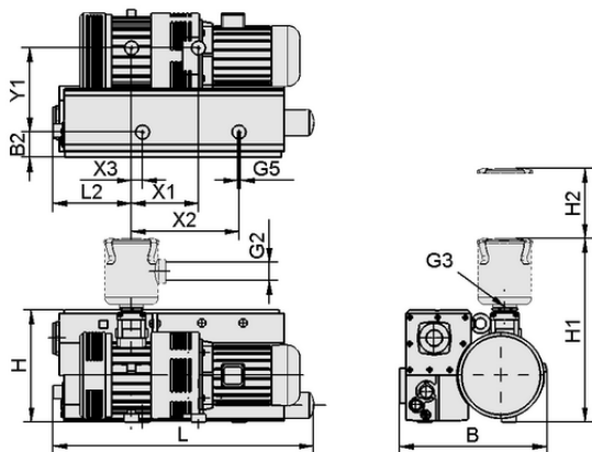
デザインデータ EVE-OG 165 AC3 F
