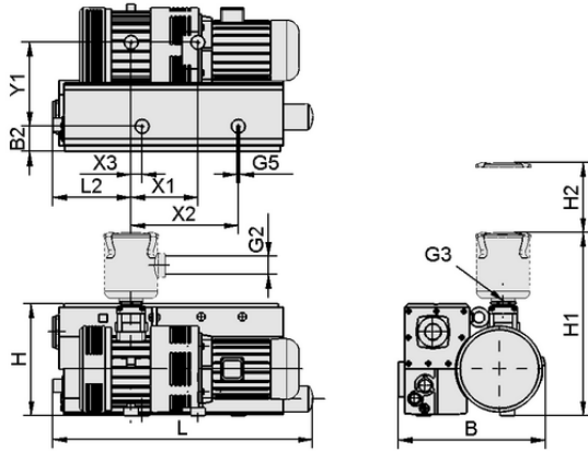
Tasarım verileri EVE-OG 165 AC3
