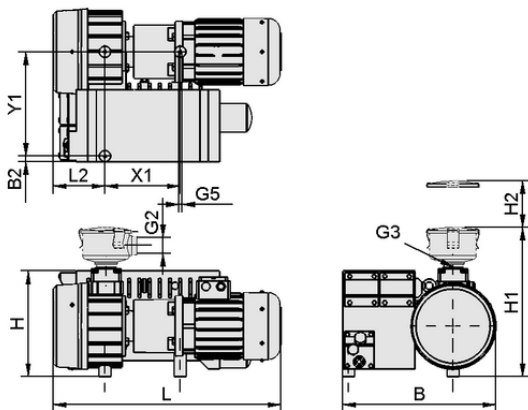
Données de construction EVE-OG 100 AC3 F
