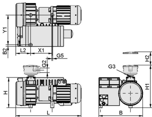
Données de construction EVE-OG 63 AC3 F
