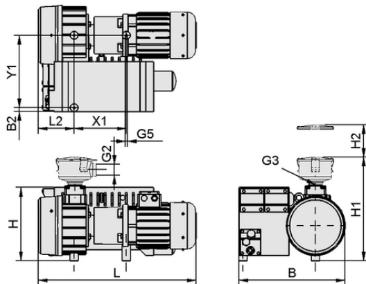
Konstruktionsdaten EVE-OG 63 AC3 F
