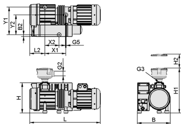
Données de construction EVE-OG 40 AC3 F
