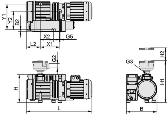
Tasarım verileri EVE-OG 40 AC3
