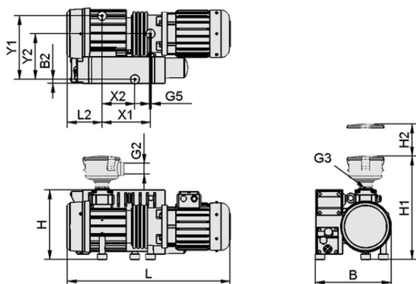
Dati di costruzione EVE-OG 25 AC3 F
