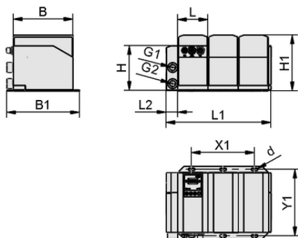
Données de construction GSPi 100 3xM12-5 24V-DC FB
