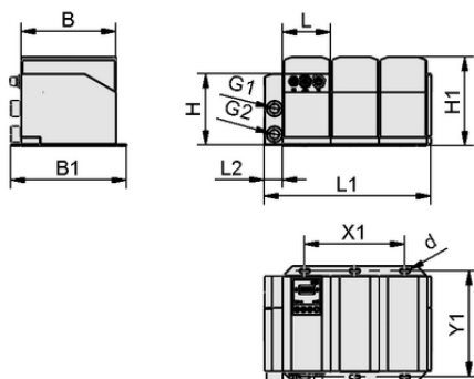
Dati di costruzione GSPc 150 2xM12-5 24V-DC FB
