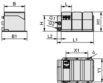
Données de construction GSPc 100 2xM12-5 24V-DC FB
