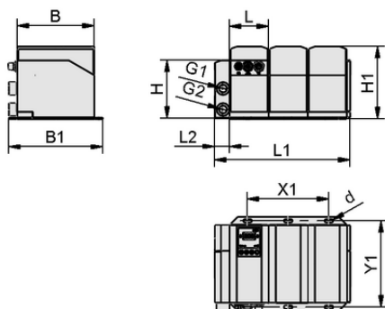
Dati di costruzione GSPc 50 2xM12-5 24V-DC FB
