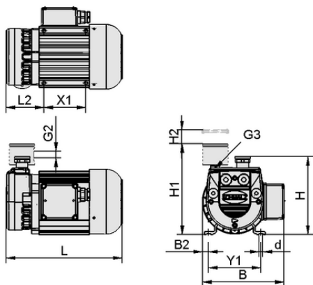
Données de construction EVE-TR 4 AC IE3-TYP1
