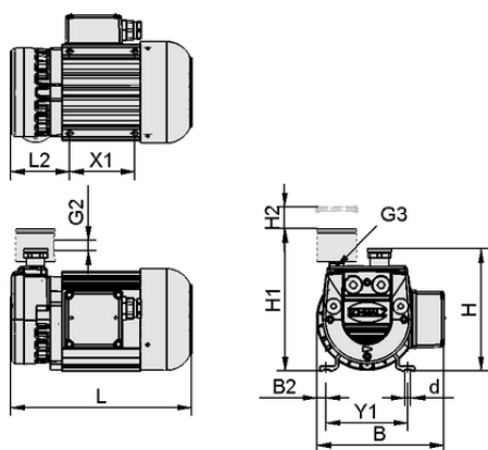
Données de construction EVE-TR 8 AC3 F
