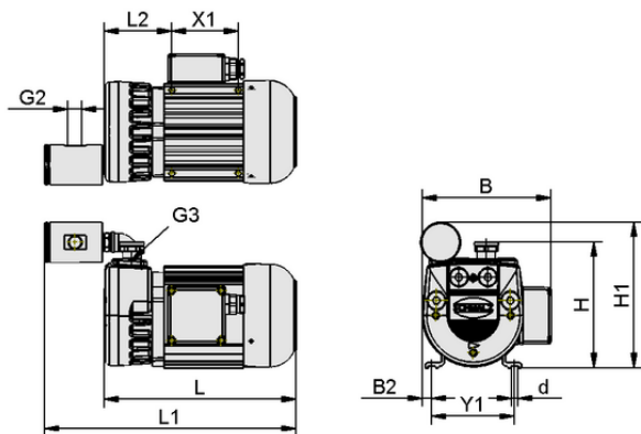
Données de construction EVE-TR 8 AC3 IE2-TYP1 F
