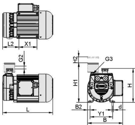
Données de construction EVE-TR 8 AC3
