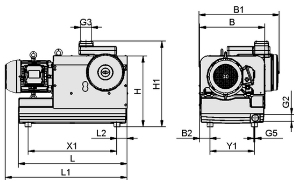
デザインデータ EVE-KL 100 AC3 IE3-TYP4 F
