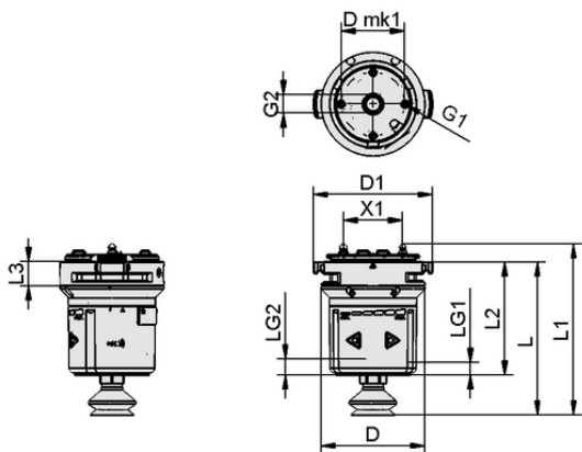
Konstruktionsdaten ECBPMi 24V-DC MATCH
