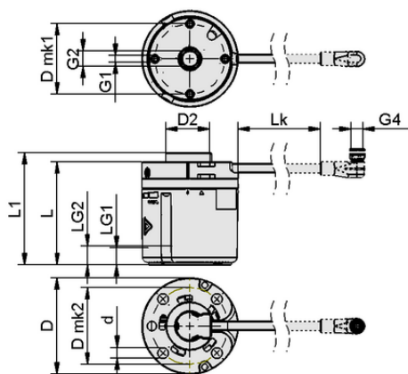
Datos de diseño ROB-SET ECBPMi FANUC
