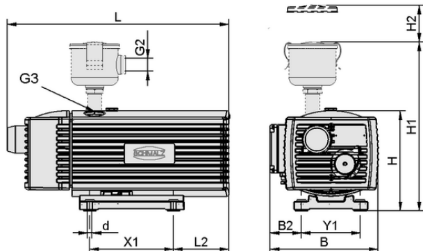
Données de construction EVE-TR 40 AC3 IE3-TYP4
