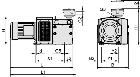
Tasarım verileri EVE-TR 80 AC3 IE3-TYP4
