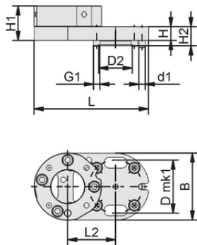
Données de construction MOD-FLAN 108x63 ECBPi
