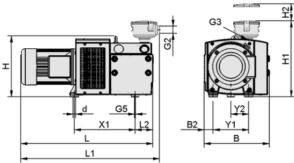
Tasarım verileri EVE-TR-X 140 AC3 IE3-TYP3 VBV
