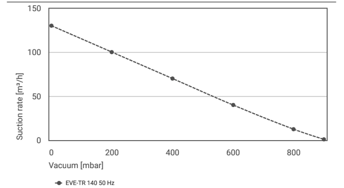
Çeşitli tahliye derecelerinde emme oranı
