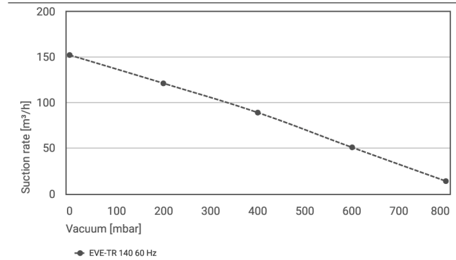
Çeşitli tahliye derecelerinde emme oranı
