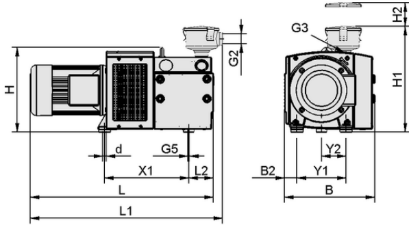
Tasarım verileri EVE-TR 100 AC3 IE3-TYP3
