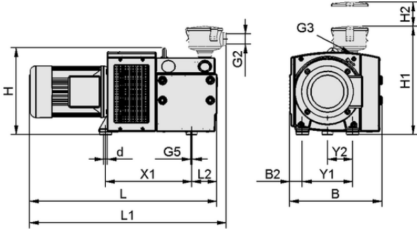
Tasarım verileri EVE-TR-X 80 AC3 IE3-TYP2 F-VB
