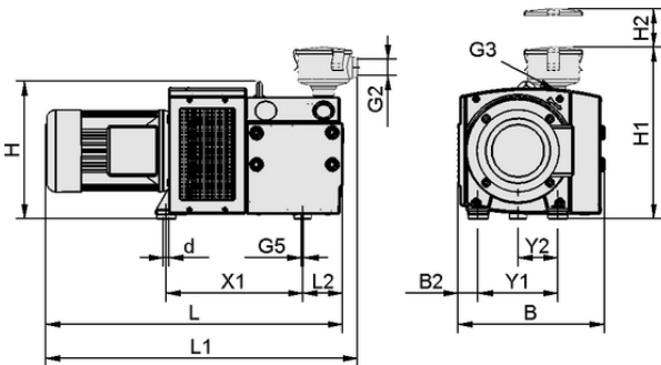
Données de construction EVE-TR 80 AC3 IE3-TYP1 F
