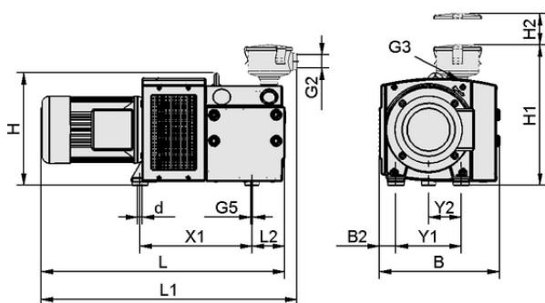
Dati di costruzione EVE-TR-X 80 AC3 IE3-TYP2 VBV
