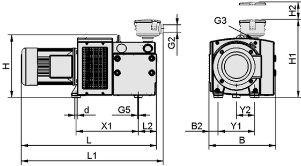
Tasarım verileri EVE-TR 140 AC3 IE3-TYP1
