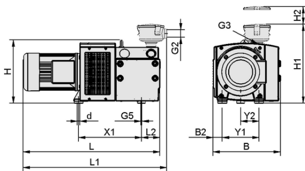
Konstruktionsdaten EVE-TR 100 AC3 IE3-TYP1
