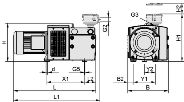
Données de construction EVE-TR 60 AC3 IE3-TYP1
