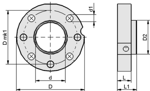
Dati di costruzione FLAN-PL UR-KUK-1
