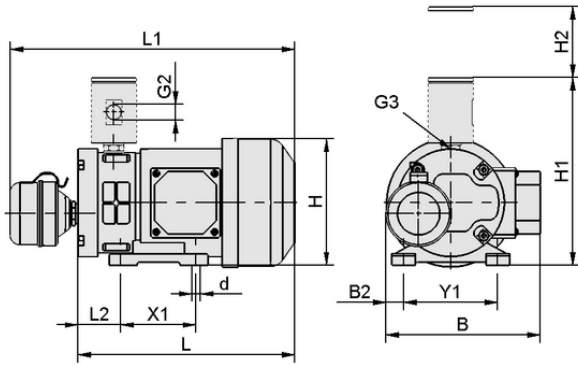
Tasarım verileri EVE-TR 8 DC
